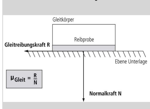
Abbildung 2 Methode zur Definition des Gleitreibungskoeffizienten
