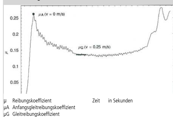
Abbildung 3 Messkurve Gleitfestigkeit einer PU-Sohle auf einem Gummibelag
